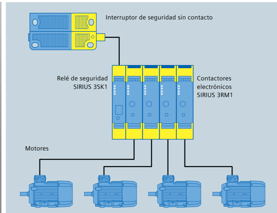
Combinación de un relé de seguridad SIRIUS 3SK1 y cuatro contactores electrónicos para la desconexión en grupo segura.
